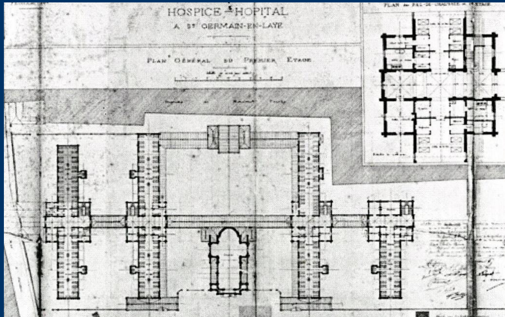
Plan du premier étage Alfred-Nicolas Normand 1884
