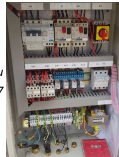
Exemple : Armoire électrique du poste Winchester - 2017
